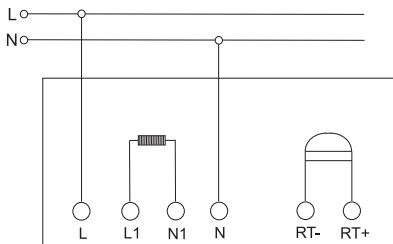
Рисунок 1 – Электрическая схема подключения термостата / Figure 1 – Electrical diagram for connecting the thermostat / 1 сурет – Термостатың жалғаудың электрлік схемасы / Figura 1 – Circuitul electric al termostatlui
