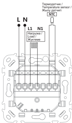
Рисунок 1 – Электрическая схема подключения / Figure 1 – Electrical diagram for connecting the backlight / 1-сурет – Жарық түсірілгішті жалғаудың электрлік схемасы
