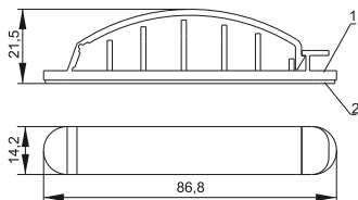
1 – изделие / product; 2 – клейкая лента / adhesive tape KC-5 / KS-5
