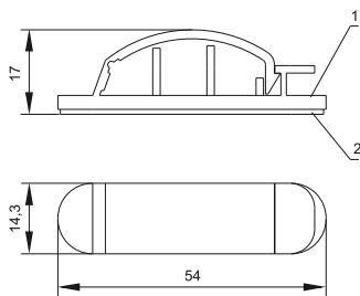
1 – изделие / product; 2 – клейкая лента / adhesive tape KC-3 / KS-3
