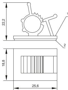
1 – изделие / product; 2 – клейкая лента / adhesive tape KC-10 / KS-10
