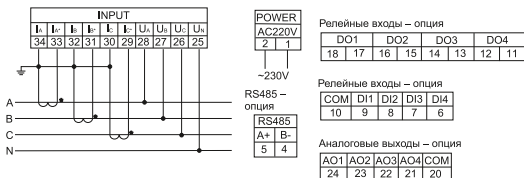
в) схема подключения мультиметра LCD к четырехпроводной сети при I > 5 A, U \leq 600 В
