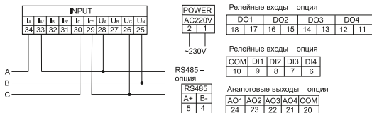
б) схема подключения мультиметра LCD к трехпроводной сети при I \leq 5 A, U \leq 600 В
