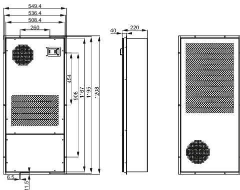
Рисунок 8 – CM-3000-230 и CM-3500-230
