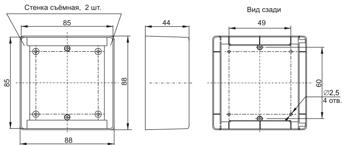
Рисунок 2 – КМКУ артикул SKK10D-U-1-KXX
