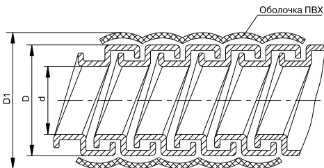
Рисунок 1 – Металлорукав типа МПГнг-LS
