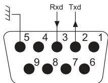
Рисунок 4 – Разъём RS-232
