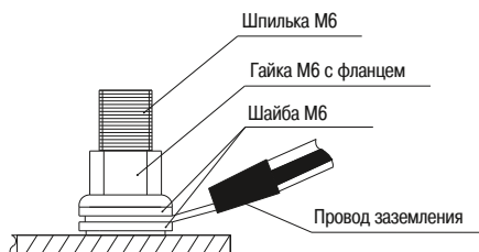
Рисунок 18 – Монтаж заземления
