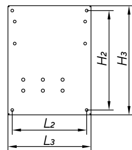
Панель монтажная
