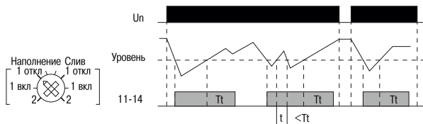
Рисунок 7 – Функциональная диаграмма реле ORL-02. Режим управления – 1 уровень (наполнение отключено)
