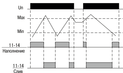
Рисунок А.5 – Функциональная диаграмма реле ORL-02. Режим управления – 2 уровня (наполнение/слив)
