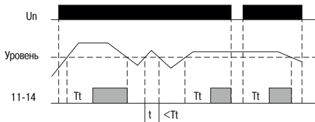
Рисунок А.8 – Функциональная диаграмма реле ORL-02. Режим управления – 1 уровень (слив включен)
