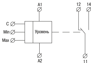
Рисунок A.2 – Схема электрическая реле Figure A.2 – Relay electrical diagram
