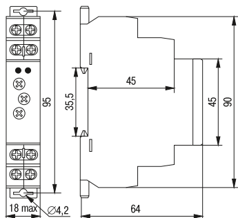
Рисунок A.1 – Габаритные и установочные размеры реле Figure A.1 – Relay overall and installation dimensions
