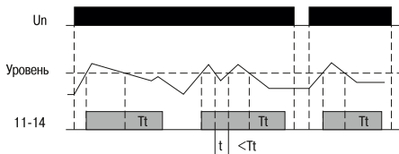
Рисунок А.9 – Функциональная диаграмма реле ORL-02. Режим управления – 1 уровень (слив отключен)
