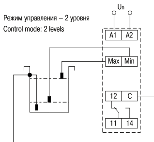
Рисунок A.3 – Схемы подключения реле Figure A.3 – Relay connection diagrams
