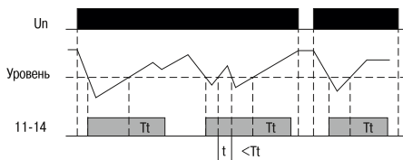
Рисунок А.7 – Функциональная диаграмма реле ORL-02. Режим управления – 1 уровень (наполнение отключено)
