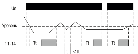
Рисунок А.6 – Функциональная диаграмма реле ORL-02. Режим управления – 1 уровень (наполнение включено)
