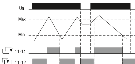
Рисунок А.4 – Функциональная диаграмма реле ORL-01. Режим управления – 2 уровня
