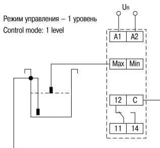
Рисунок A.2 – Схема электрическая реле Figure A.2 – Relay electrical diagram
