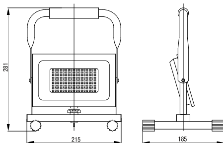
Рисунок 2 – СДО 06-50П
