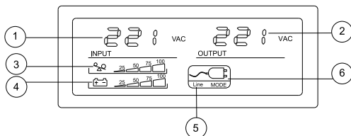
Рисунок 3 – Дисплей ИБП
