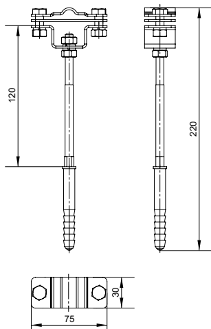
Рисунок / Figure 1 – Габаритные размеры / Overall dimensions
