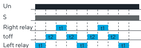
Диаграмма работы реле
