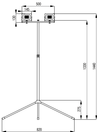
Рисунок 1 – СДО 06-2×30Ш
