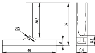
Рисунок 3 – Габаритные и установочные размеры держателя маркировки
