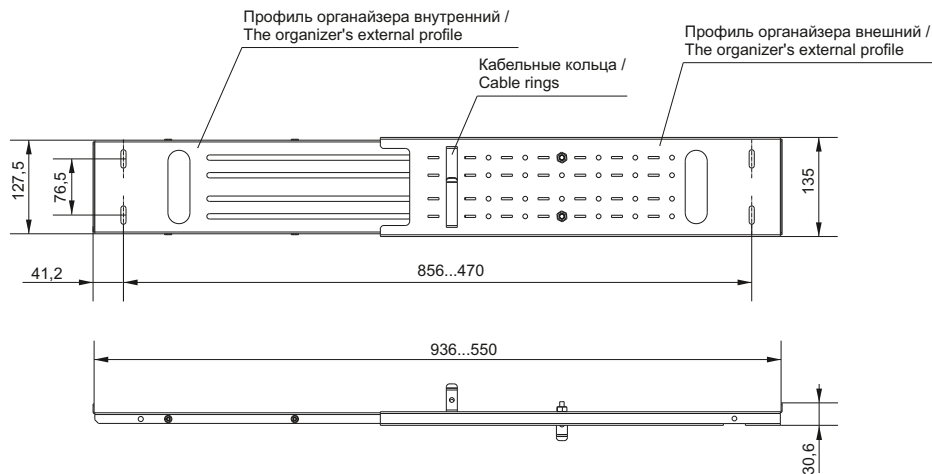
Рисунок 2 – Органайзер кабельный горизонтальный / Figure 2 – Horizontal cable organizer
