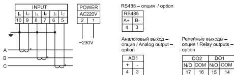
б) схема подключения 3-ф. амперметра при I > 5 A / connection diagram of 3-ph. ammeter at I > 5 A
