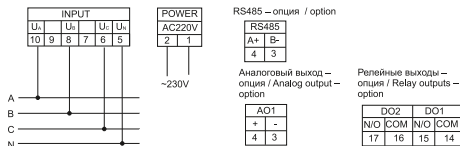
в) схема подключения 3-ф. вольтметра для измерения фазного напряжения при U \leq 600 V / connection diagram of 3-ph. voltmeter for measuring phase voltage at U \leq 600 V
