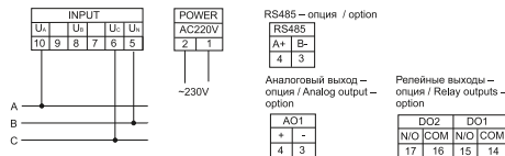
г) схема подключения 3-ф. вольтметра для измерения фазного напряжения при U > 600 V / connection diagram of 3-ph. voltmeter for measuring phase voltage at U > 600 V
