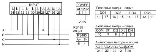
а) схема подключения мультиметра LCD к четырехпроводной сети при I \leq 5 A, U \leq 600 В
