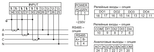
с) схема подключения мультиметра LCD к четырехпроводной сети при I > 5 A, U \leq 600 В
