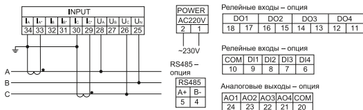
д) схема подключения мультиметра LCD к трехпроводной сети при I > 5 A, U \leq 600 В
