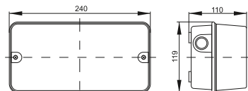
Рисунок 3 – Габаритные и установочные размеры светильника НПП3006
