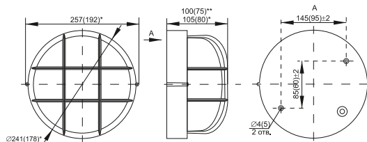
Рисунок 1 – Габаритные и установочные размеры светильников НПП1102, НПП1107
