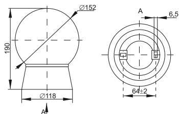
Рисунок 4 – Габаритные и установочные размеры светильника НПП 9101
