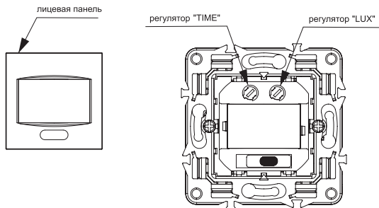
Рисунок 1 – Конструкция датчика
