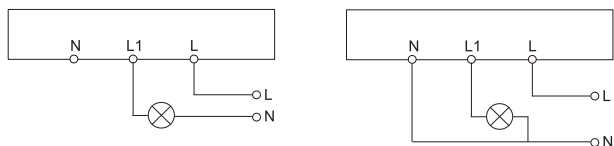
Рисунок 2 – Электрические схемы подключения датчика
