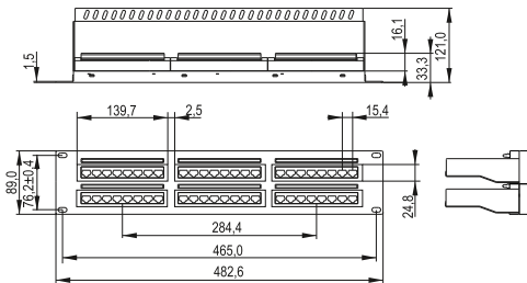
Рисунок 8 – PP48-2UC5EU-D05-1
