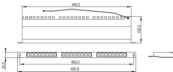
Рисунок 5 – PP24-D05UC5ES-D05H
