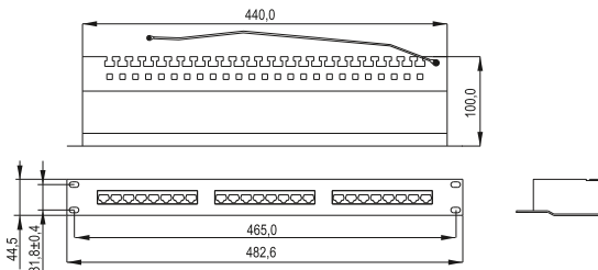
Рисунок 6 – PP24-1UC5ES-D05
