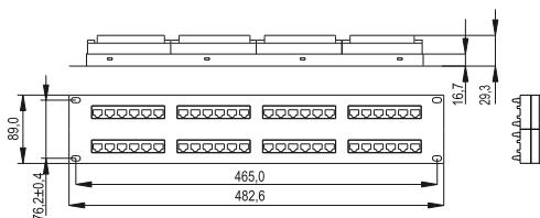
Рисунок 4 – PP48-2UC5EU-D05, PP48-2UC5EU-D05L
