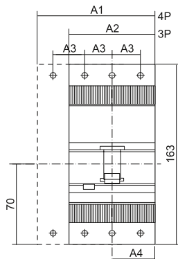
Шаблон разметки установочных отверстий ПМ1/П-32(33)
