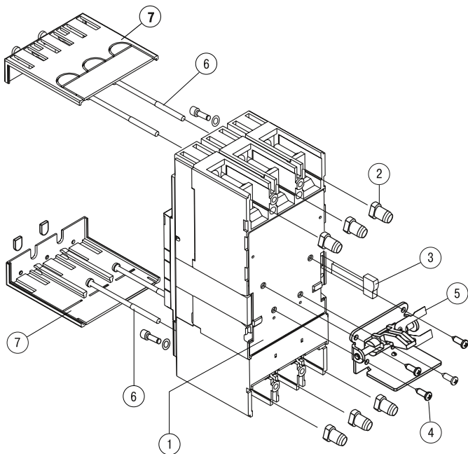
Рисунок 36 Схема сборки тыльных панелей ПМ1/П-35(37), ПМ1/Р-35(37)
