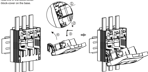
Рисунок 6 – Монтаж горизонтальных ПБП на токи 250–630 А / Figure 6 – Installation of horizontal PVR for 250–630 A currents
