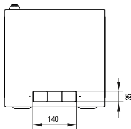
Рисунок 1 – Габаритные и установочные размеры шкафа / Figure 1 – Overall and installation dimensions of the cabinet / 1 – şuret – Şkaftyñ gabarittık jãne ornatu õlşemder / Рисунок 1 – Габаритні та установчі розміри шафи
