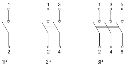
Рисунок 2 – Схемы электрические выключателя
