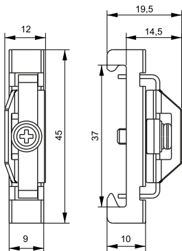
Рисунок 1 – Габаритные размеры ограничителей
