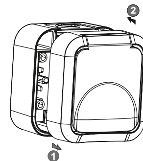
Рисунок 1 – Порядок монтажа розетки / Figure 1 – Socket installation procedure / 1 сурет – Розетканы монтаждау тәртібі
