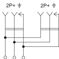
б) Розетка двухместная с заземляющим контактом горизонтальная / Horizontal two-gang socket-outlet with ground contact / Жерге тұйықтау контактісі бар көлденең екі орындық розетка
