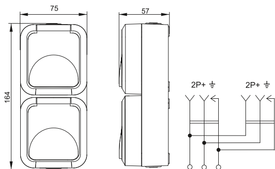
в) Розетка двухместная с заземляющим контактом вертикальная / Vertical two-gang socket-outlet with ground contact / Жерге тұйықтау контактісі бар тік екі орындық розетка
