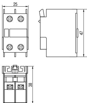
Рисунок 1 Габаритные размеры ПКИ-11, ПКИ-20
