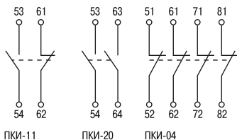
Рисунок 3. Электрические схемы ПКИ
