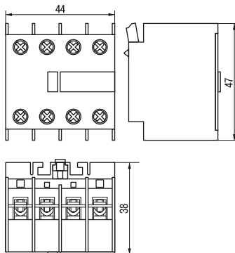
Рисунок 2 Габаритные размеры ПКИ-04, ПКИ-22, ПКИ-40
