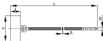
а) хомут типа ХП1
