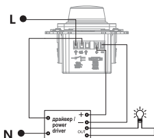
a) FI-D24-0200-X* (обычный / conventional / тұрақты)
