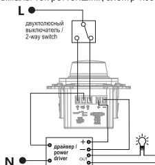
b) FI-D20-0200-P-X* (проходной / pass-through / өтпелі)
