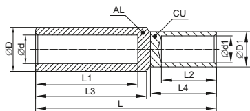
Рисунок 1. Гильзы медноалюминиевые, внешний вид и габаритные размеры.
