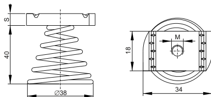
Рисунок 2 – STRUT-болт с конусной пружиной / Figure 2 - STRUT bolt with conical spring / Сурет 2 – STRUT- конусты серіппелі бұраңда
