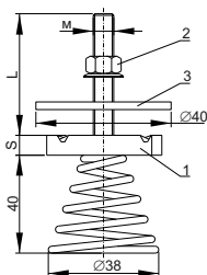
Рисунок 4 – Комплект для STRUT-профиля / Figure 4 – Kit for STRUT profile / Сурет 4 – STRUT- профильге арналған жиынтық
