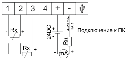
Рисунок 1 – Схема подключения преобразователя
