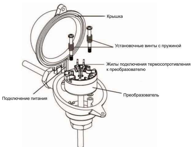
Рисунок 1 – Схема подключения преобразователя
