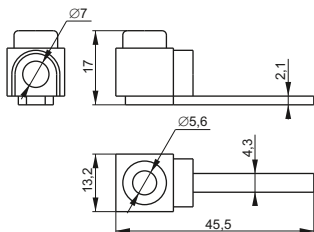
Рисунок 1 – Габаритные и установочные размеры клеммы KBM 4–25 мм 2 (удлиненная) / Figure1 – Overall and mounting dimensions of the KVM 4–25 mm 2 terminal (longish) / 1-suret – KVM 4–25 mm 2 klemmasynyn gabarittik jäne ornatu ölçemderi (üzartylğan) / Рисунок 1 – Габаритні та установчі розміри клеми KBM 4–25 мм 2 (подовжена)
