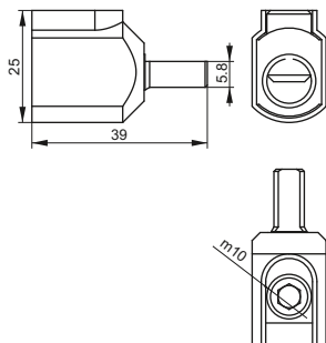
Рисунок 2 – Габаритные и установочные размеры клеммы KBM 16–50 мм 2 / Figure1 – Overall and mounting dimensions of the KVM 4–25 mm 2 terminal (longish) / 2-suret – KVM 16–50 mm 2 klemmasynyn gabarittik jäne ornatu ölçemderi / Рисунок 2 – Габаритні та установчі розміри клеми KBM 16–50 мм 2
