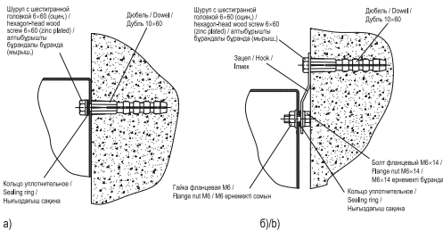
Рисунок / Figure / Сурет 2 – Крепление корпуса к
