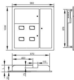
Рисунок / Figure / Сурет 1 – Корпус на 2–6 квартир / Enclosure for 2–6 apartments / 2–6 пәтерге арналған корпус
