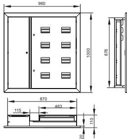
Рисунок / Figure / Сурет 4 – Корпус на 7 и 8 квартир (слаботочный отсек слева) / Enclosure for 7 and 8 apartments (ELV compartment is from left side) / 7 және 8 пәтерге арналған корпус (сол жағында әлсіз тоқты бөлік)
