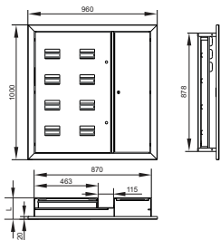
Рисунок / Figure / Сурет 2 – Корпус на 7 и 8 квартир / Enclosure for 7 and 8 apartments / 7 және 8 пәтерге арналған корпус
