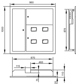
Рисунок / Figure / Сурет 3 – Корпус на 2–6 квартир (слаботочный отсек слева) / Enclosure for 2–6 apartments (ELV compartment is from left side) / 2–6 пәтерге арналған корпус (сол жақта әлсіз тоқты бөлік)
