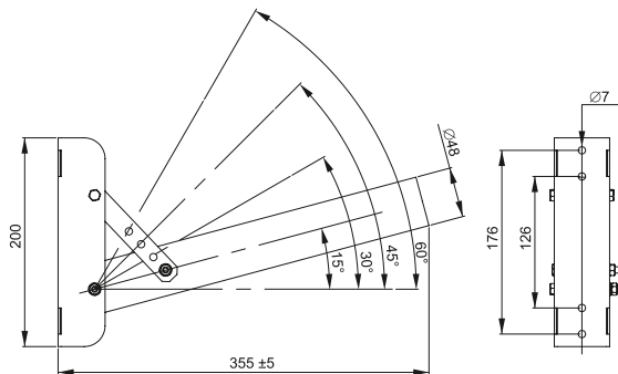
Рисунок 5 – Кронштейн LDKU0D-CR-48-0350-23-K01
