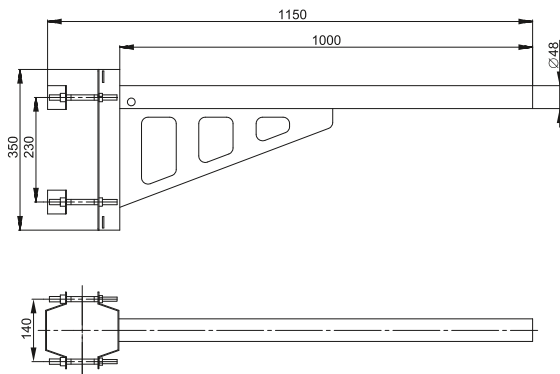
Рисунок 8 – Кронштейн LDKU0D-CR-48-1000-12-K03
