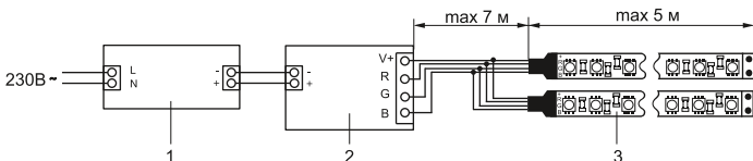
1 – блок питания; 2 – RGB контроллер; 3 – RGB светодиодная лента
