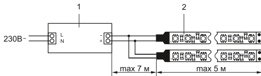
1 – блок питания; 2 – светодиодная лента
