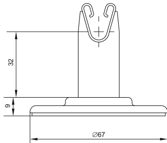
Рисунок 1 – Габаритные размеры держателя / Figure 1 – Overall dimensions of the Holder / 1 сурет – Ұстатқыштың жалпы өлшемдері
