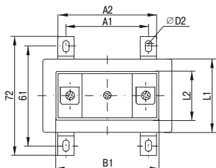
а) модификации ТТИ-30 габарит 1, ТТИ-40, ТТИ-60, ТТИ-85, ТТИ-100, ТТИ-125
