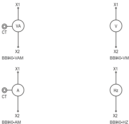
Рисунок 1 – Схемы подключения индикаторов / Figure 1 – Indicator connection diagrams
