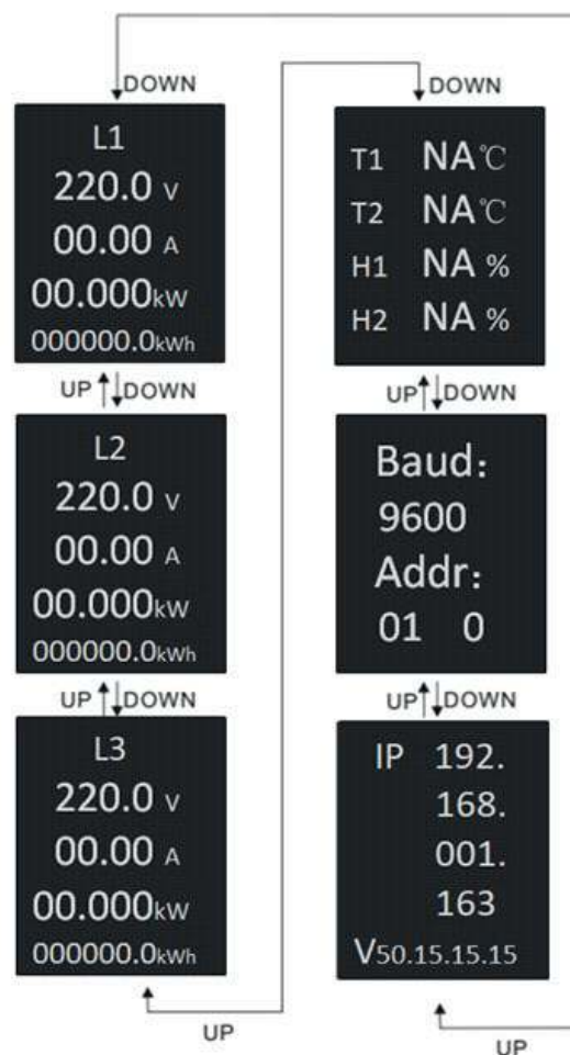
Рисунок 9 – Просмотр значения текущих параметров
