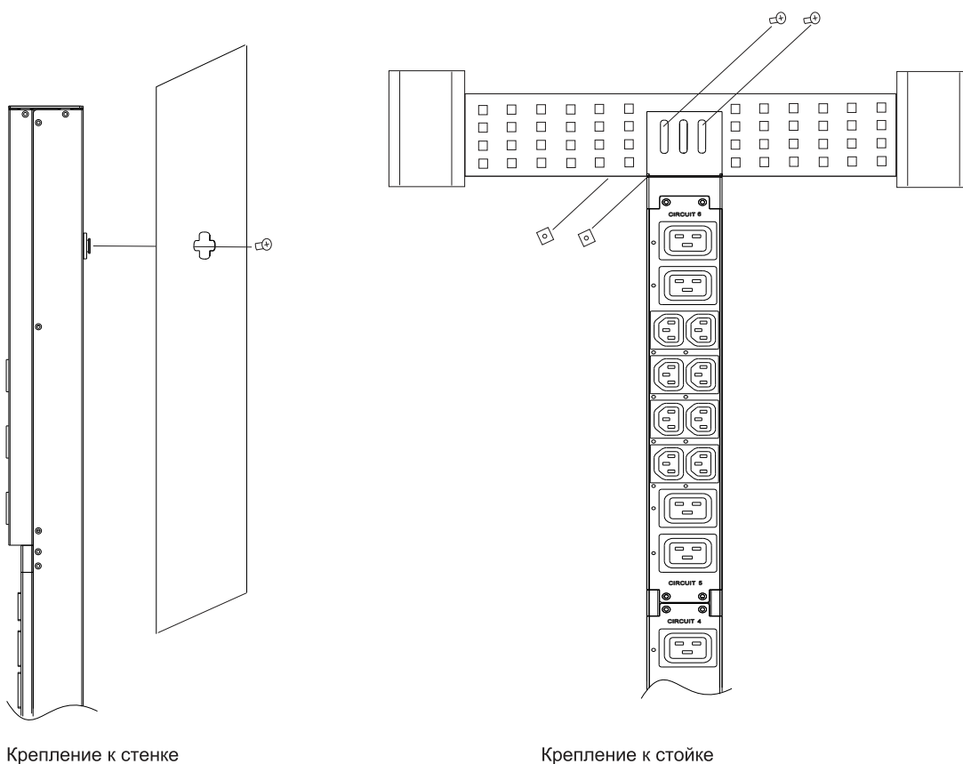
Рисунок 7 – Монтаж блока в вертикальном положении
