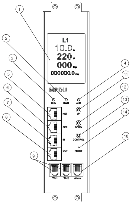
Рисунок 8 – Панель управления
