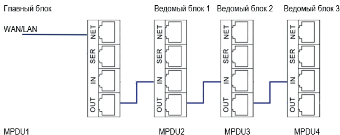
Рисунок 11 – Схема соединения
