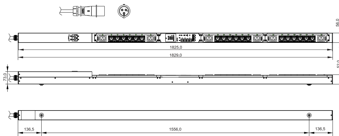
Рисунок 2 – AN-PM13-24-18C13-06C19-41, CN-PM23-24-18C13-06C19-41, AN-PM33-24-18C13-06C19-41, CN-PM43-24-18C13-06C19-41
