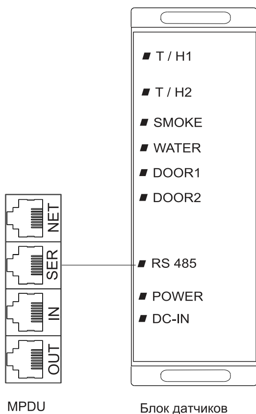
Рисунок 14 – Подключение блока датчиков
