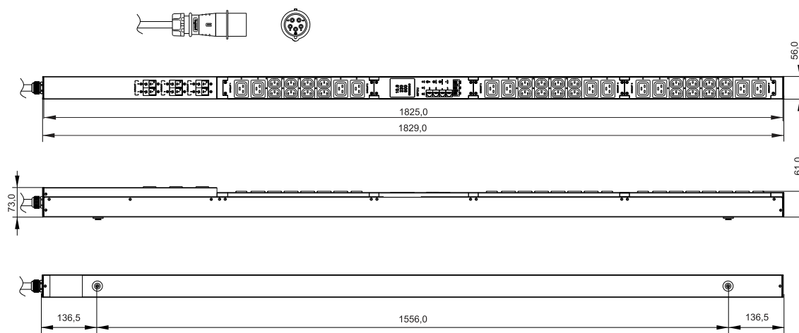
Рисунок 5 – AN-PM13-36-24C13-12C19-43, CN-PM23-36-24C13-12C19-43, AN-PM33-36-24C13-12C19-43, CN-PM43-36-24C13-12C19-43
