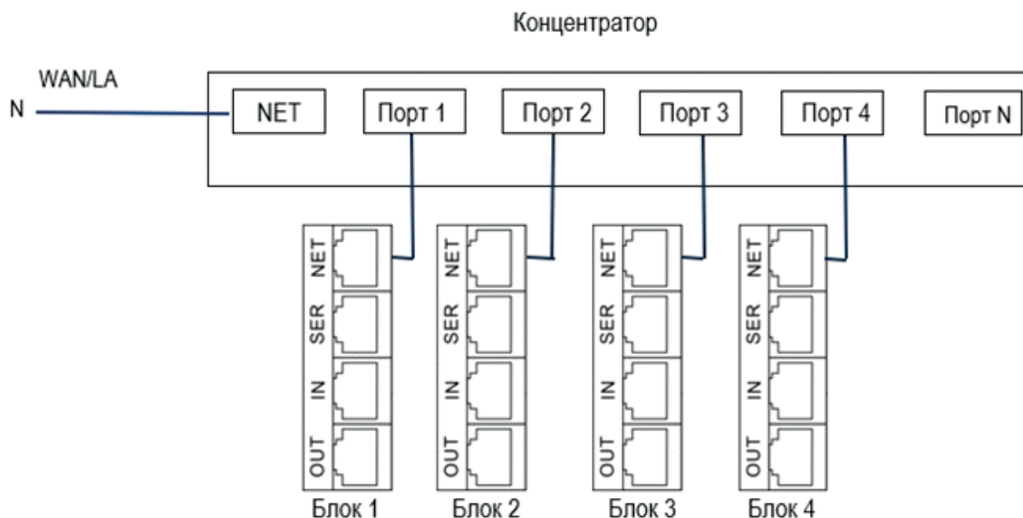
Рисунок 12 – Схема подключения «звезда»
