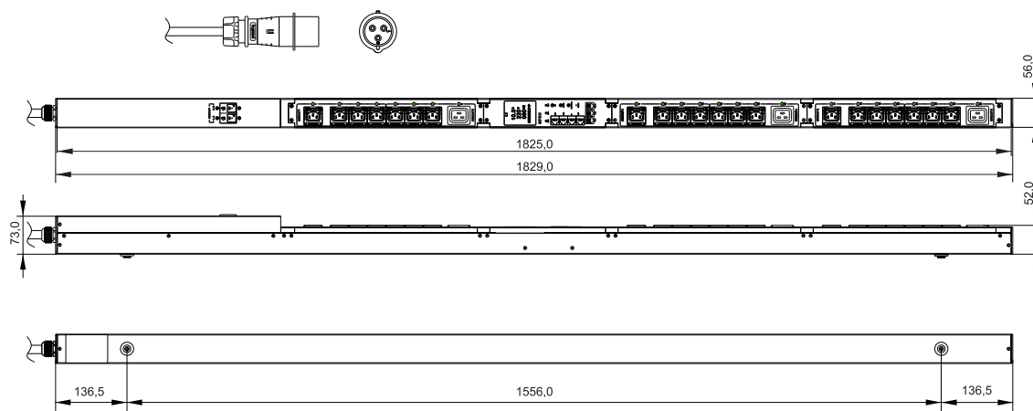
Рисунок 3 – AN-PM13-24-21C13-03C19-41, CN-PM23-24-21C13-03C19-41, AN-PM33-24-21C13-03C19-41, CN-PM43-24-21C13-03C19-41
