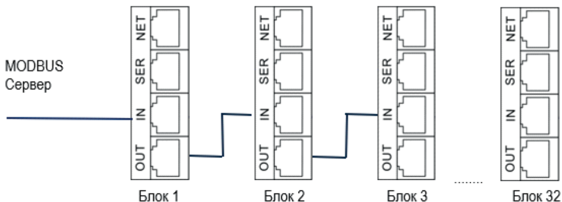
Рисунок 13 – Схема последовательного соединения для протокола Modbus-RTU
