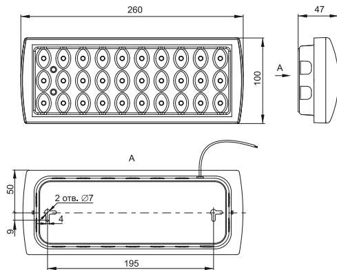
Рисунок 1 – ДПА 2101
