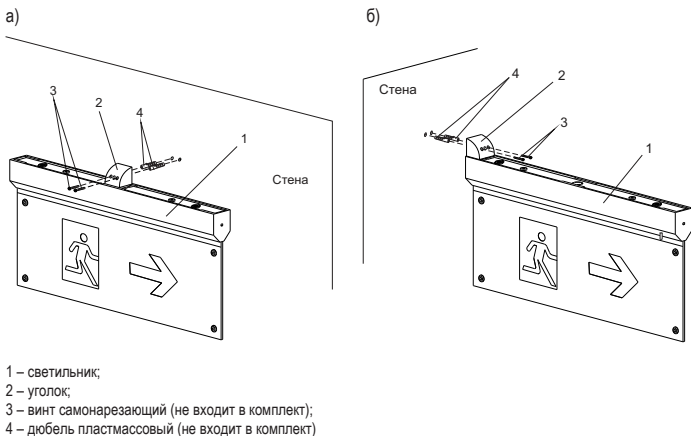
Рисунок 3 – Монтаж накладной
